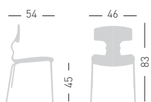
TOLO NA Techno polymer shell, 4-Legged chromed frame Scocca in tecnopolimero multi-colore, telaio in metallo cromato.
