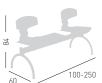
TOLO GM Techno polymer shell, grey painted bench frame. Scocca in tecnopolimero multi-colore, telaio panca verniciato grigio.
