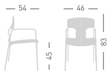
TOLO TB Techno polymer shell, 4-Legged chromed frame with armrests. Scocca in tecnopolimero multi-colore, telaio in metallo cromato con braccioli.
